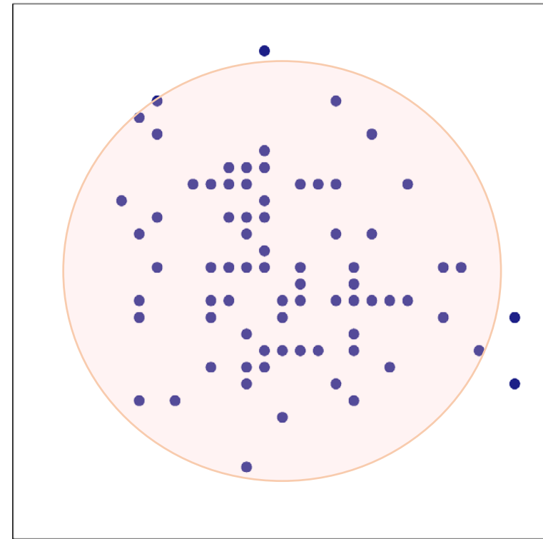
|r_{xy}| \approx 0 : 無相関
